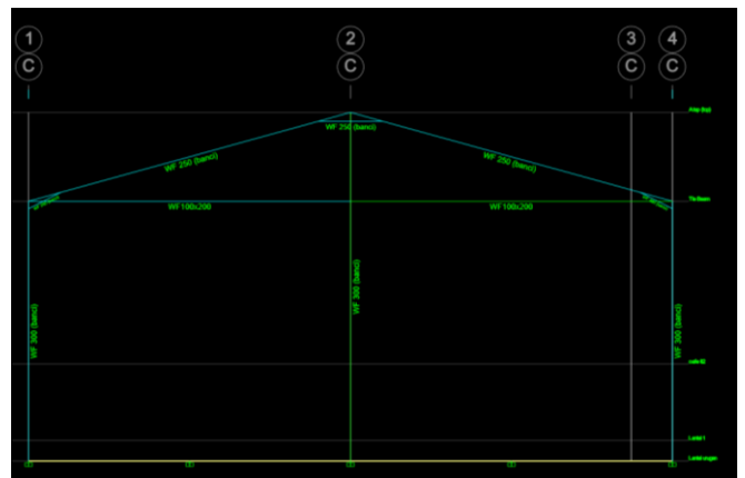
Gambar 12. Hasil Unity Check dalam ETABS untuk Potongan C – C
