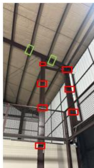
Gambar 14. Penambahan Plat Stiffener di kolom dalam dengan jarak antar plat 150 cm
