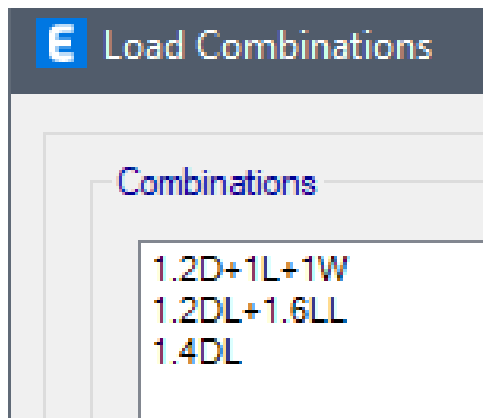
Gambar 9. Kombinasi Beban yang Dimasukkan Dalam ETABS
