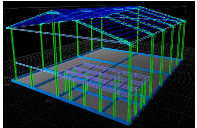
Gambar 8. Gambar Lapangan dari Aplikasi ETABS
